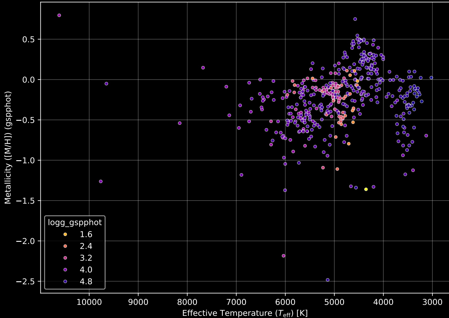
APOGEE DR17 Field: [200+45] Stellar Population Parameters (n= 463)
